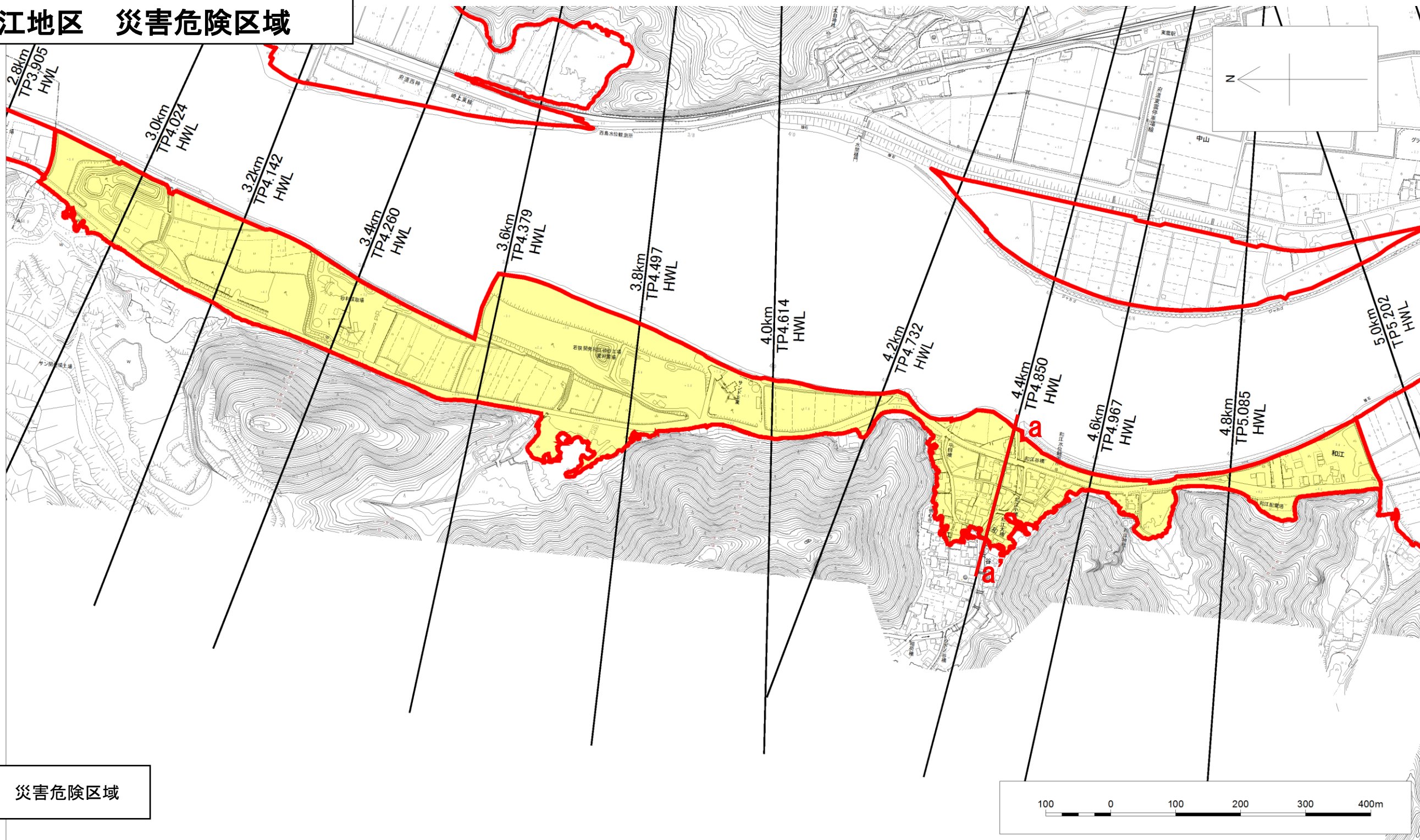
横断面 (4.4km付近) a-a'
