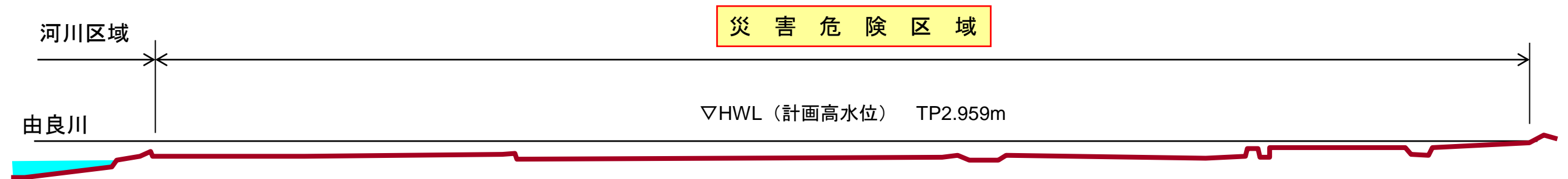
横断図 (1.2km付近) a-a'
