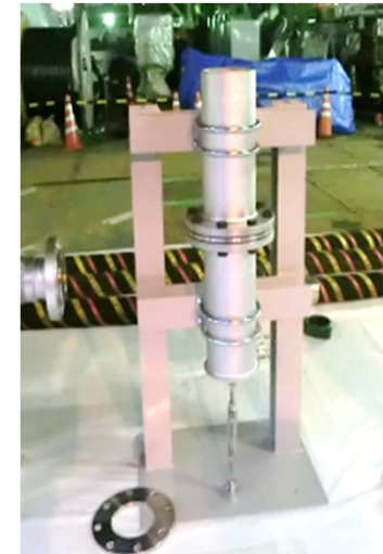
大容量ポンプ海水系統～冷却水系統 接続閉止板入替訓練設備
