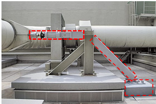
配管補強の例
