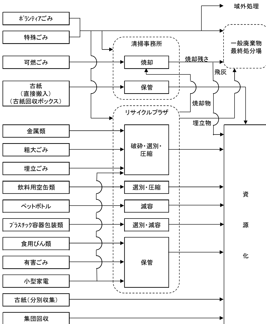
図 6-1 ごみ処理フロー
